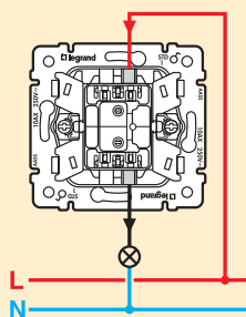
Обикновен ключ
