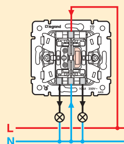
Сериен ключ с индикатор при включено положение
