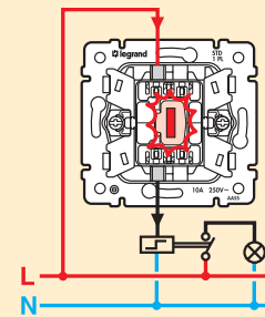
Единичен ключ за контролиране на реле със символ на лампа
