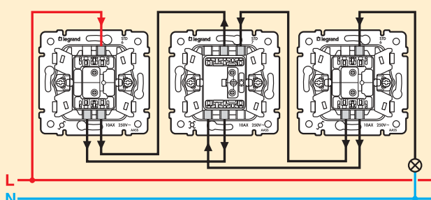
Кръстат ключ
