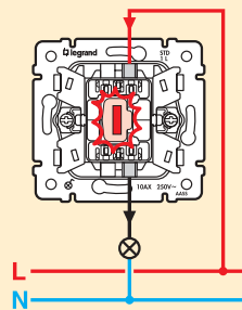
Ключ със светлинна индикация
