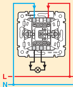
Двуполусен ключ
