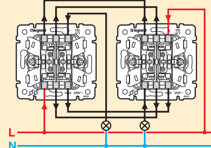
Сериен дивидаторен ключ
