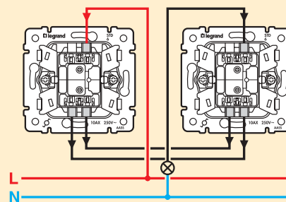
Дивиаторен ключ
