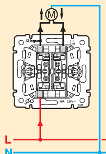
Ключ за управление на щори
