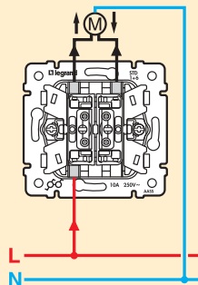
Бутон за управление на щори
