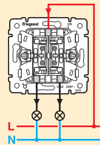
Сериен ключ
