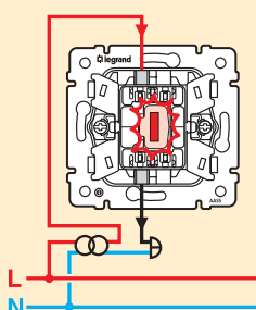
Бутон за звънец със светлинна индикация
