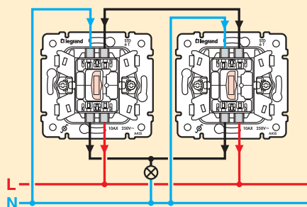
Дивиаторен ключ с индикатор при включено положение
