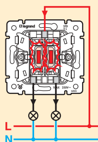
Сериен ключ със светлинна индикация
