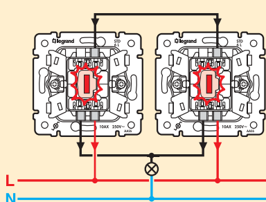
Дивиаторен ключ със светлинна индикация
